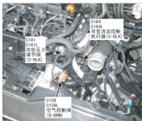
28. 发动机前左
