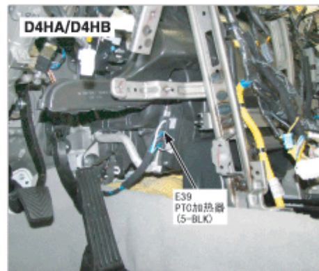
27. 仪表板中央
