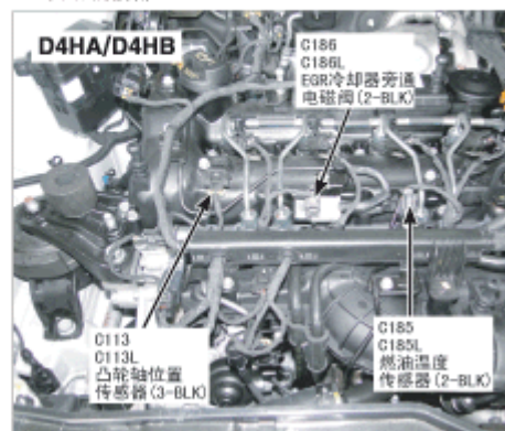
30. 发动机前部
